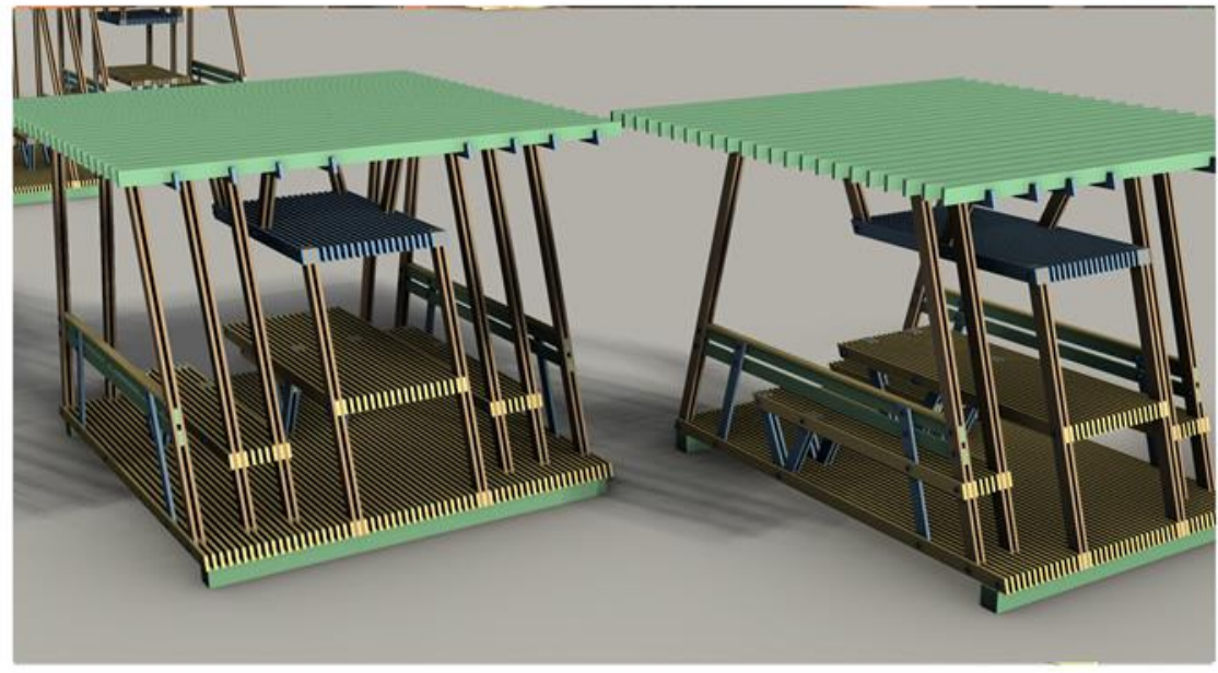
Теневые пляжные беседки в комбинации со столами и скамейками
